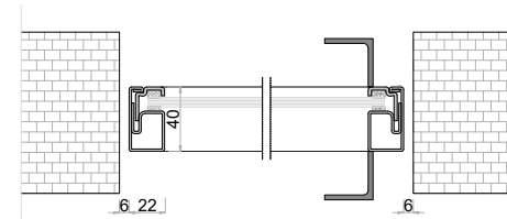
DE | Einzeltür Pivot EN | Single Pivot Door
