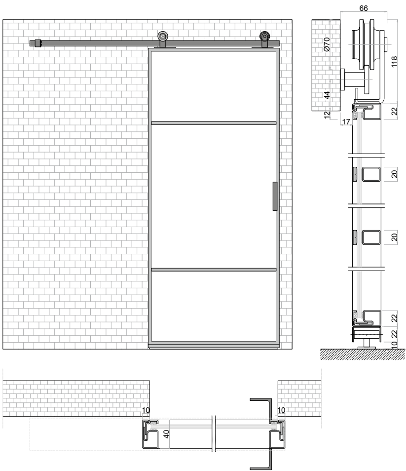
DE | Einzelschiebetür EN | Single Sliding Door
