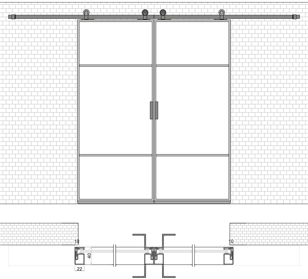
DE | Doppelschiebetür EN | Double Sliding Door
