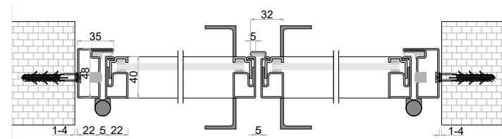
DE | Doppeltür EN | Double Door
